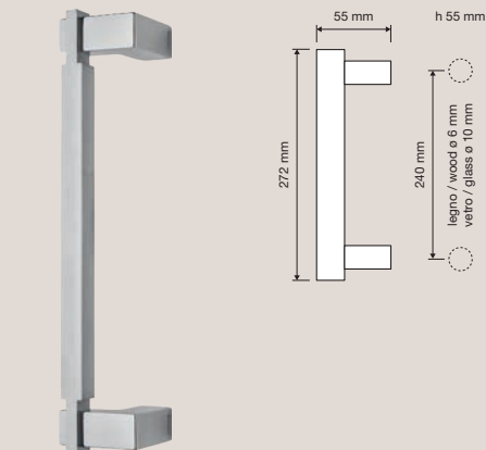
1050 MZ 240 Maniglione zancato. Interassi disponibili 240-320-440-500- 800. / Offset pull handle. Available distances 240-320- 440-500-800.
