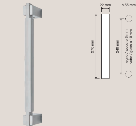
1050 MN 240 Maniglione. Interassi disponibili 240-320- 440-500-800. / Pull handle. Available distances 240-320- 440-500-800.
