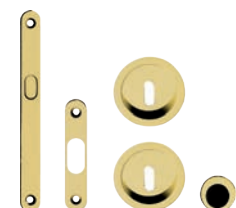
332 KT Kit incasso tondo foro chiave con maniglia trascinamento, serratura e chiave / Round inset handle kit key hole with finger pull, locking system and key
