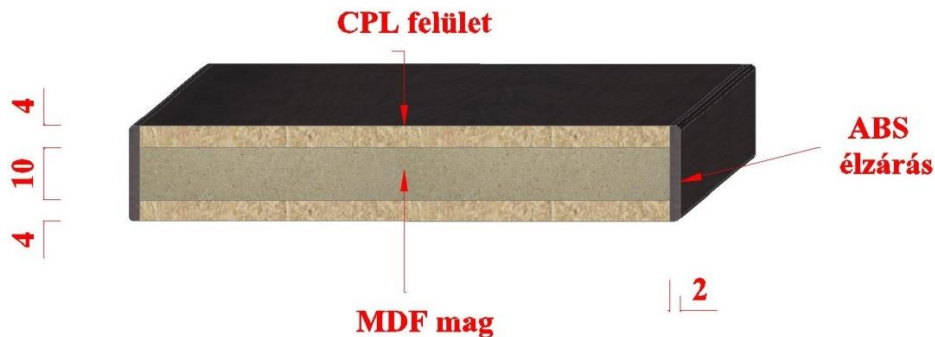
Színazonos CPL küszöb szerkezeti felépítése
