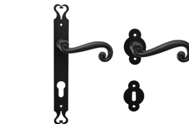
/// készleten SERRANO hosszúcímes és díszes rozettás F fekete A fogantyú: zamak / cím: vas M A=105 mm B=250 mm C=30 mm D=50 mm
