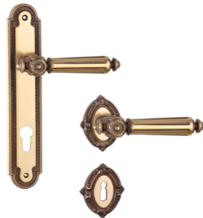
/// készleten WIEN hosszúcímes/rozettás F antik A réz M A=135 mm B=240 mm C=45 mm D=55x68 mm
